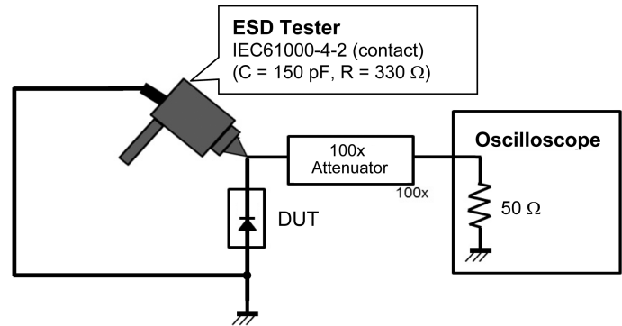
Fig. 6.1.3 IEC61000-4-2 (Contact)
