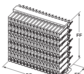
Receptacle (Backplane)
