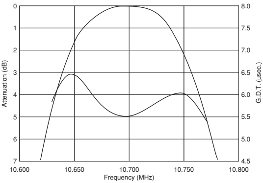
SFELF10M7KAH0-B0
