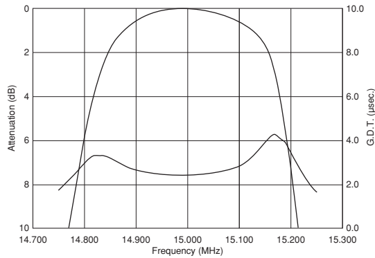
SFECV15M0EQ0001-R0
