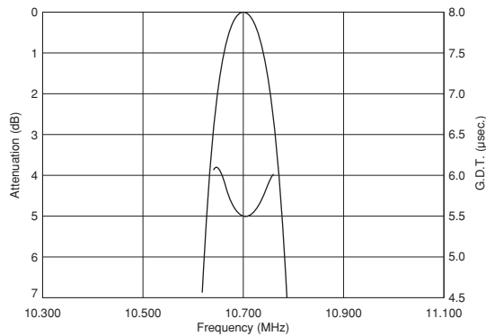
SFECV10M7JA00-R0
