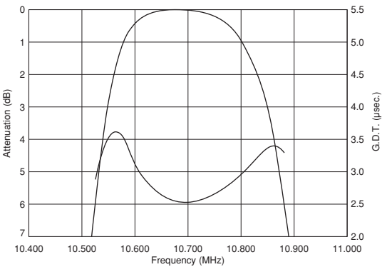
SFELF10M7FA0G-B0
