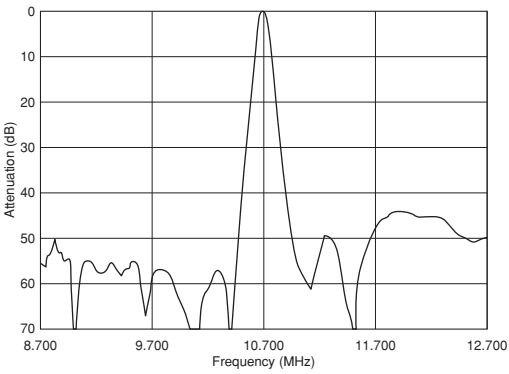
SFELF10M7LFTA-B0
