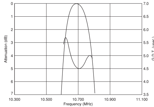
SFECV10M7KA00-R0
