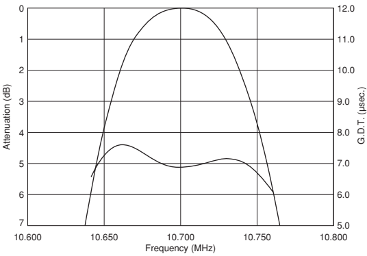
SFELF10M7LFTA-B0
