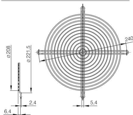
78128-2-4039 Fan size 200
