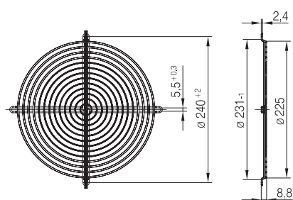
35138-2-4039 Fan size 208
