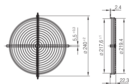
35139-2-4039 Fan size 208
